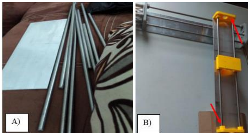
Figura 19. A) Husillos y guías de 8mm radio x 50cm, B) Soportes para las guías lineales, 2 por eje. Junto con guías lineales de 50 cm de largo.
