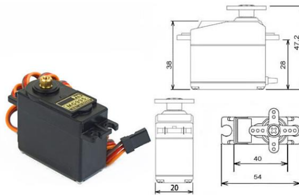
Figura 28. Servomotor MG955 utilizado en el robot cartesiano para el accionamiento del elemento terminal. 25
