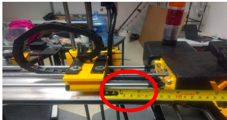
Figura 54. Desplazamiento eje Y
