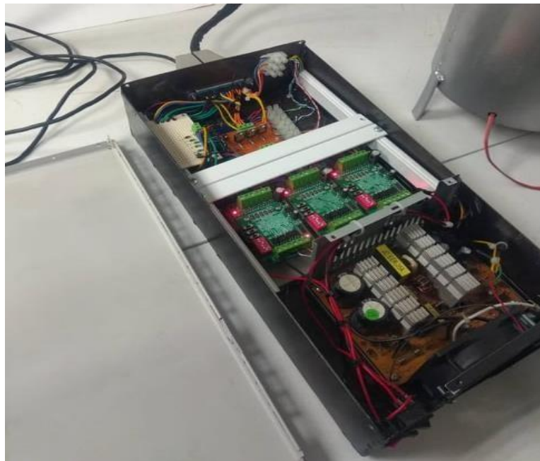
Figura 43. Se ilustra la caja de control con todos sus componentes soldados y ruteados.
